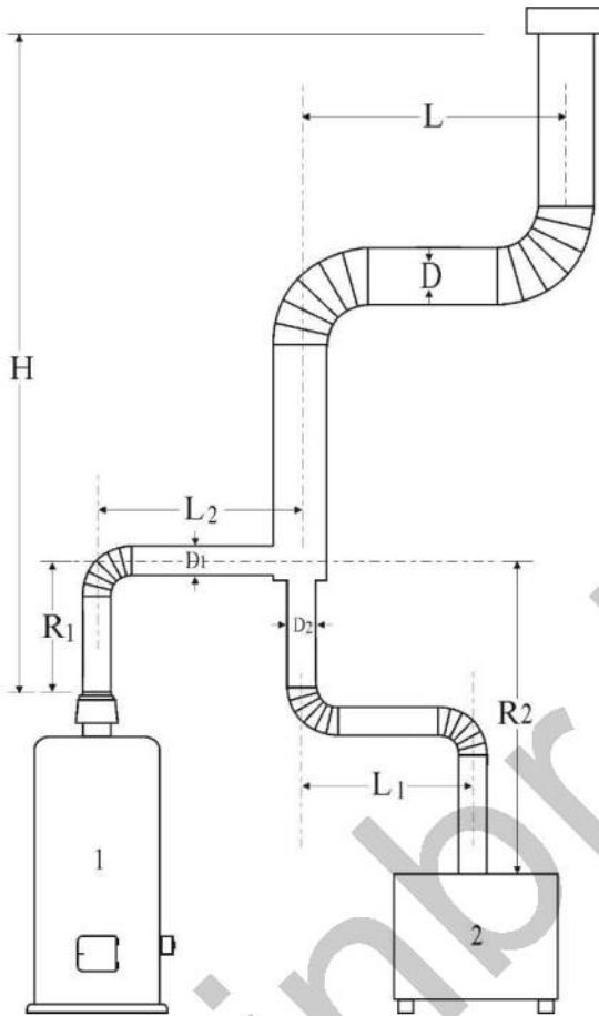
شکل ۱۷-۷-۲ دودکش برای دو یا چند دستگاه گازسوز که در یک طبقه نصب شده‌اند
